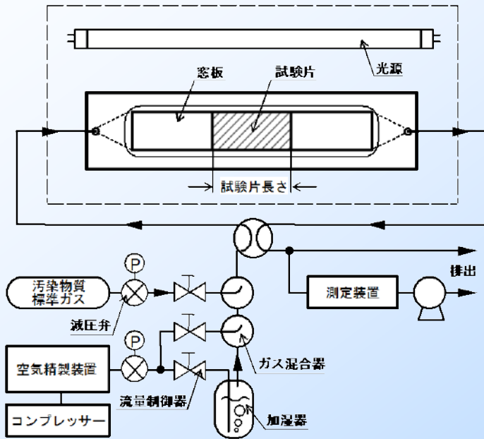
試験装置
